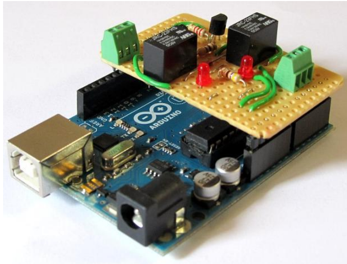
รูปที่ 1.12 ตัวอย่างการต่อใช้งาน Arduino บนบอร์ด Shield ที่สร้างขึ้นเอง (ที่มา www.Chokelive.com/blog/2013/07/Micro-Controller-Application.html )
