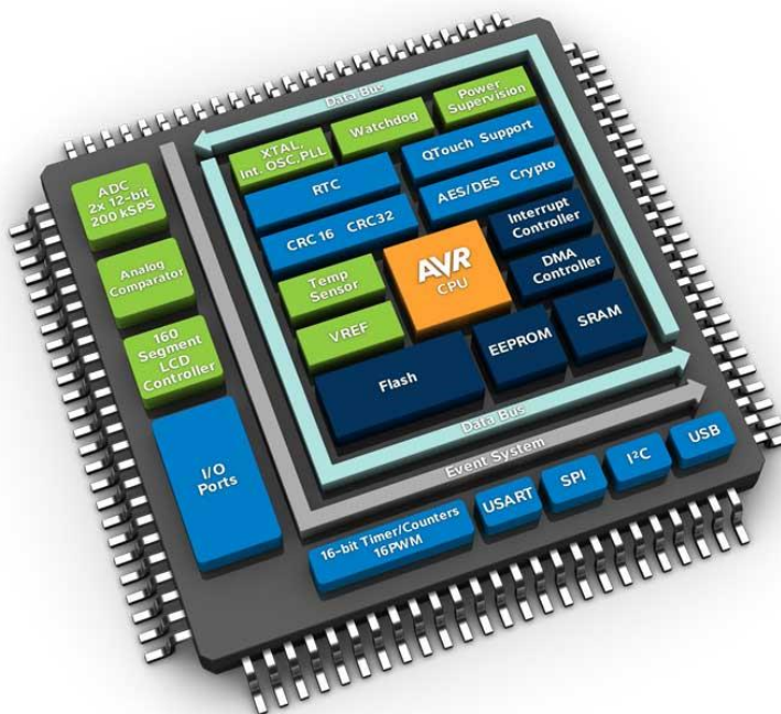
รูปที่ 1.15 สถาปัตยกรรมภายในไมโครคอนโทรลเลอร์ AVR
