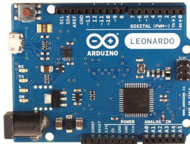
รูปที่ 1.21 ไมโครคอนโทรลเลอร์ Arduino Leonardo (ที่มา www.Thaieasyelec.com )
