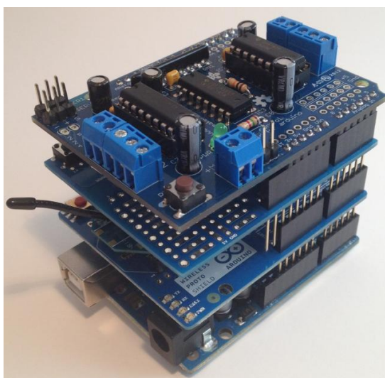
รูปที่ 1.11 ตัวอย่างการต่อใช้งาน Arduino บนบอร์ด Shield สำเร็จรูป
