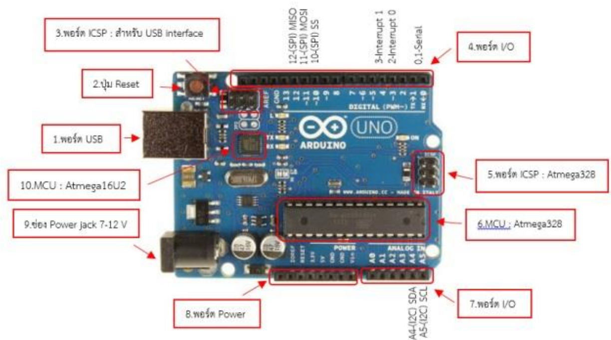
รูปที่ 1.17 ไมโครคอนโทรลเลอร์ Arduino Uno R3
