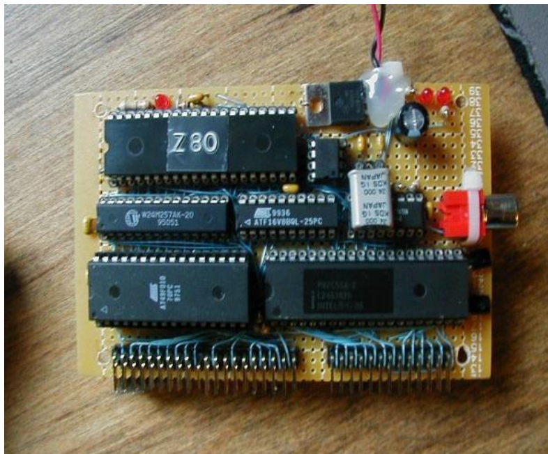
รูปที่ 1.3 ตัวอย่างการใช้งาน Z-80 บนบอร์ดทดลองจริง
