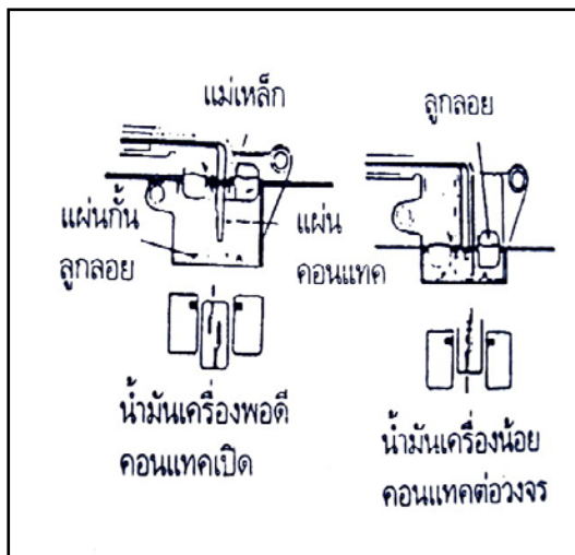
รูปที่ 5.6 คอนแทคเปิดแต่ต่อวงจร
