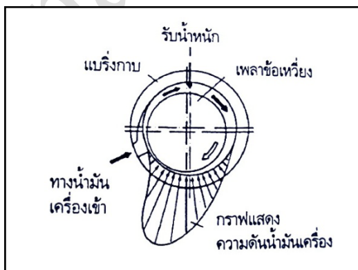
รูปที่ 5.1 ความดันน้ำมันเครื่องที่หล่อลื่นเพลลา
