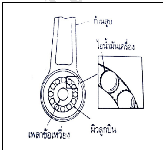
รูปที่ 5.12 ก้านสูบใช้กับลูกปืน ต้องการหล่อลื่นด้วยใส่น้ำมันเครื่อง
